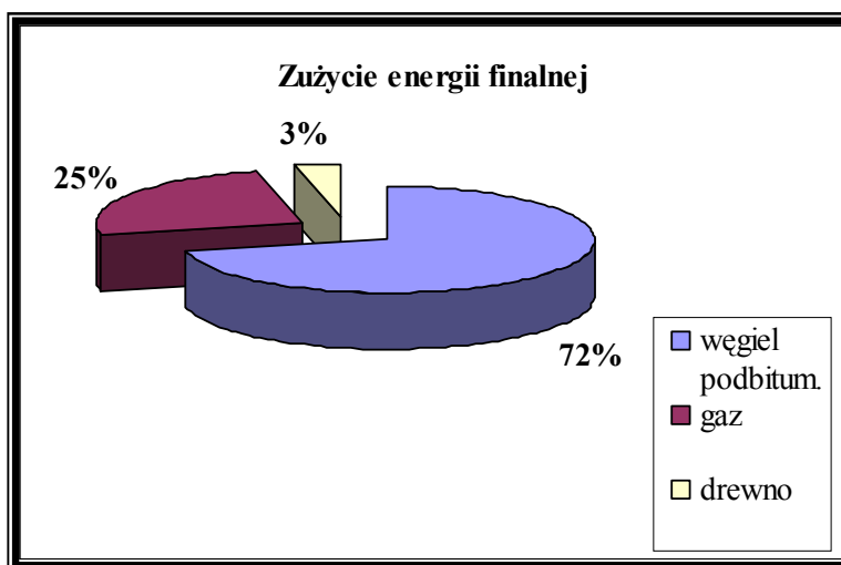
Rysunek 6. Struktura zużycia energii finalnej w obiektach usługowo-przemysłowych w 2014 r.
